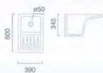
101 lavadero lava-roupa laundry sink bac à laver
