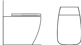
Inodoro p/depósito alto / Sanita à parede T3163 - 56x35.5cm
