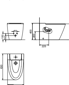
Alimentación encastada Alimentation encastrée Built-in water feed
